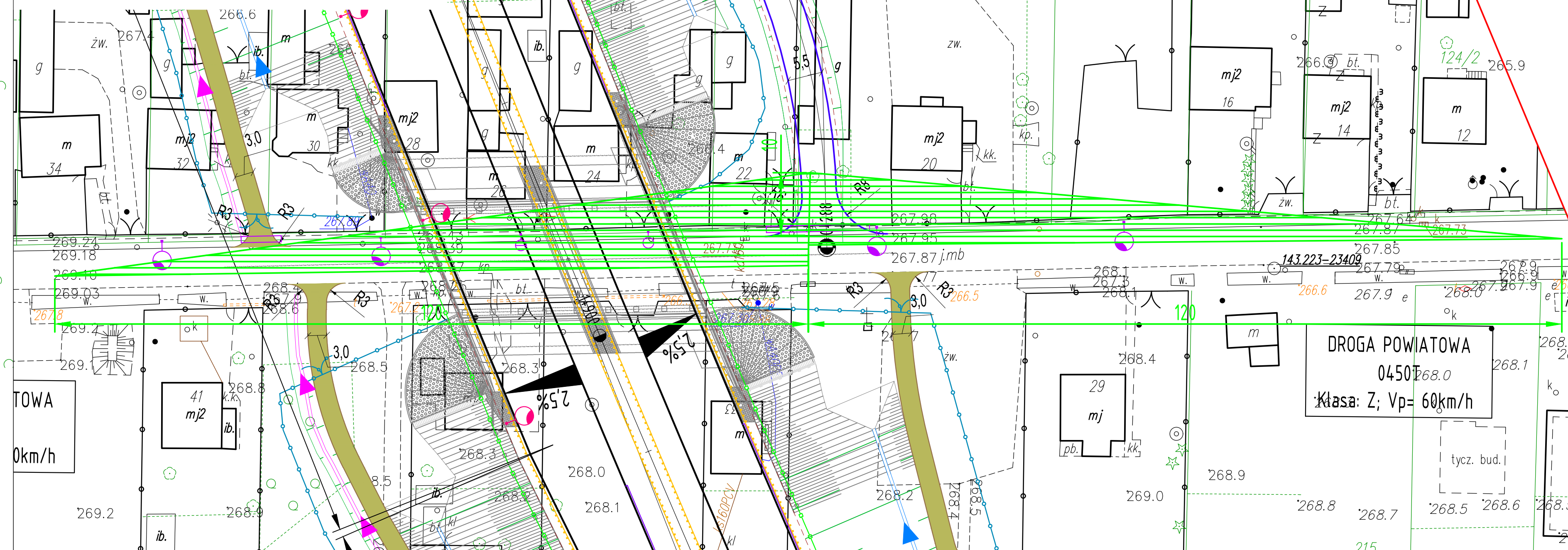
Skrzyżowanie DJ2 z DP0450T
