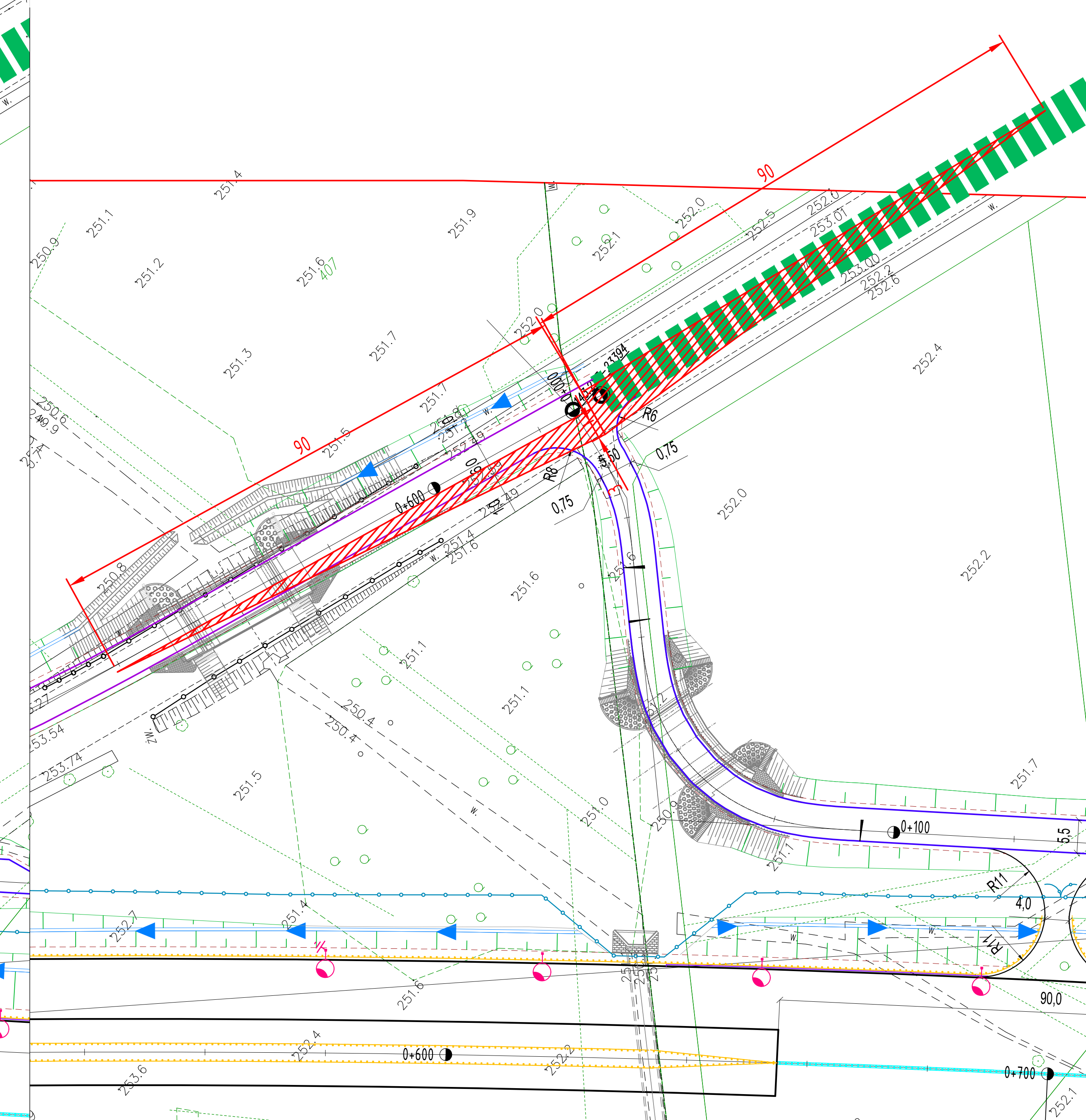
Skrzyżowanie DJ1 z DP0491T
