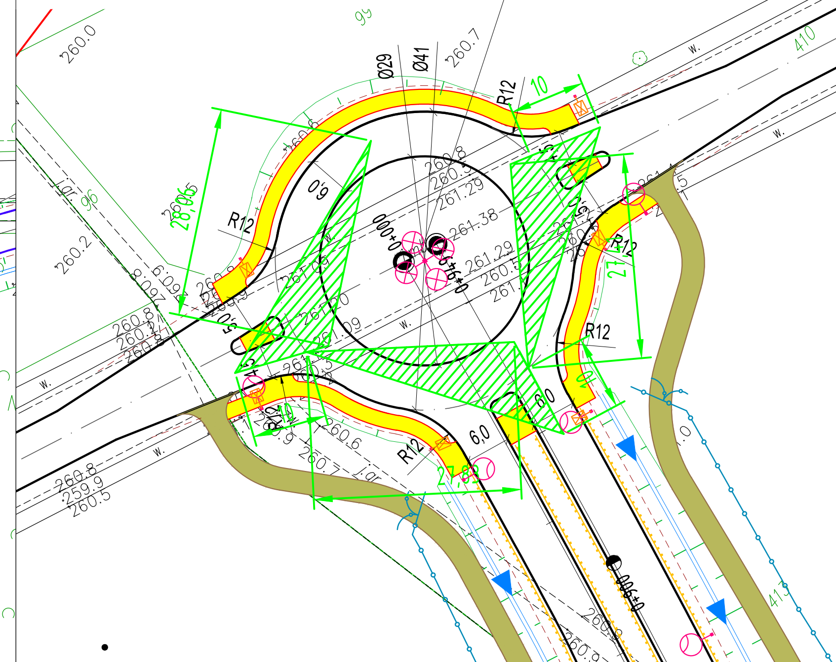
Rondo węzeł "Mniów"
