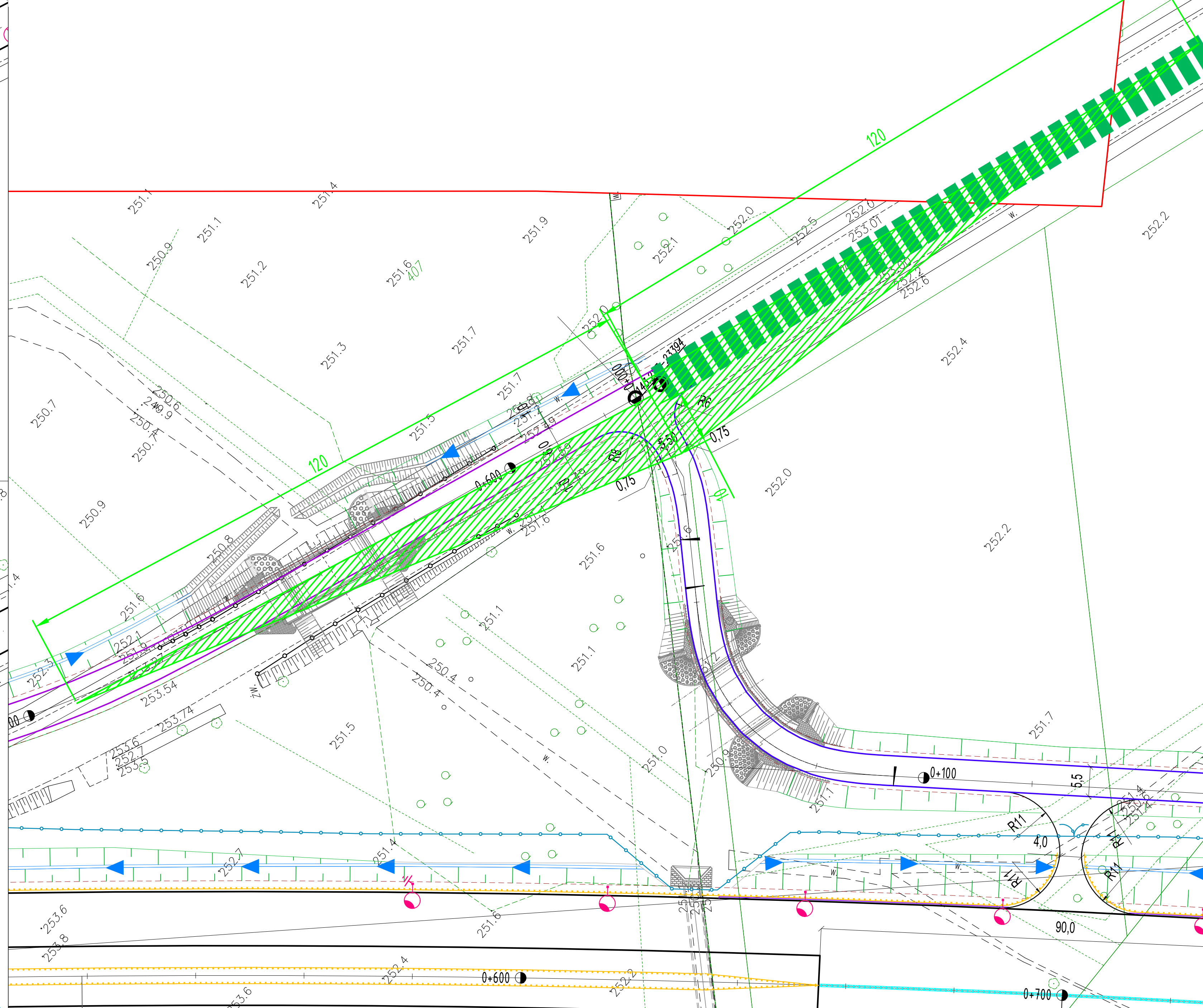
Skrzyżowanie DJ2 z DP0450T
