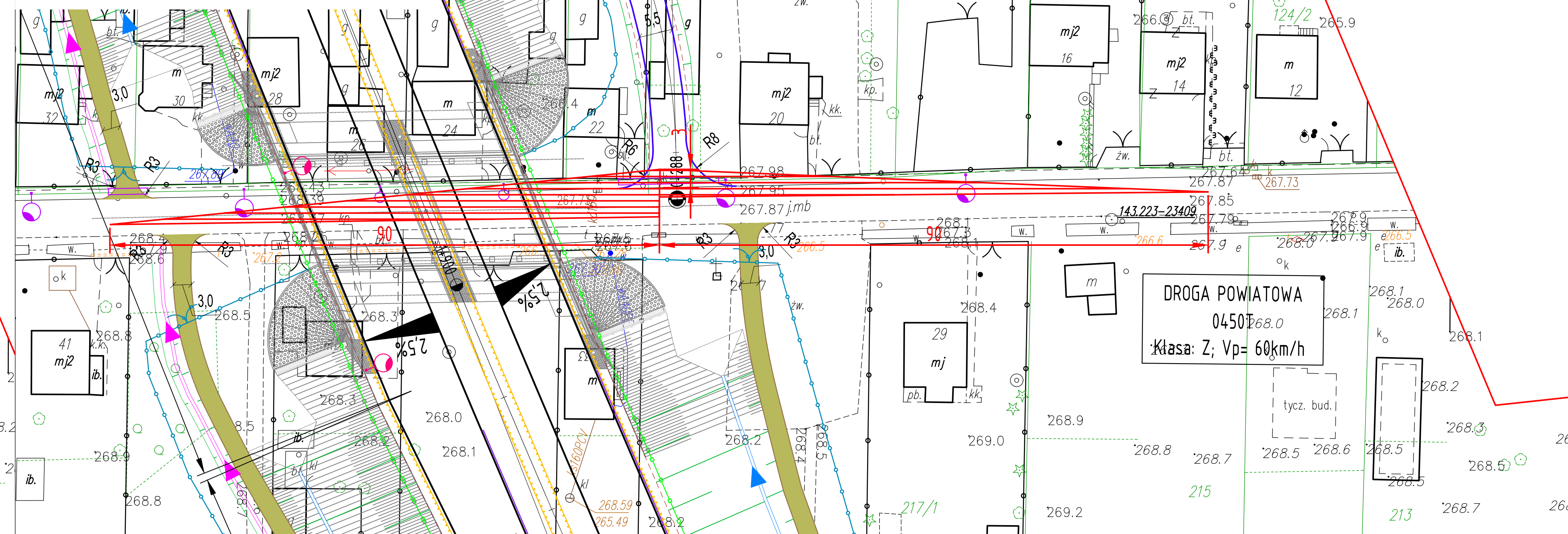
Skrzyżowanie DJ2 z DP0450T
