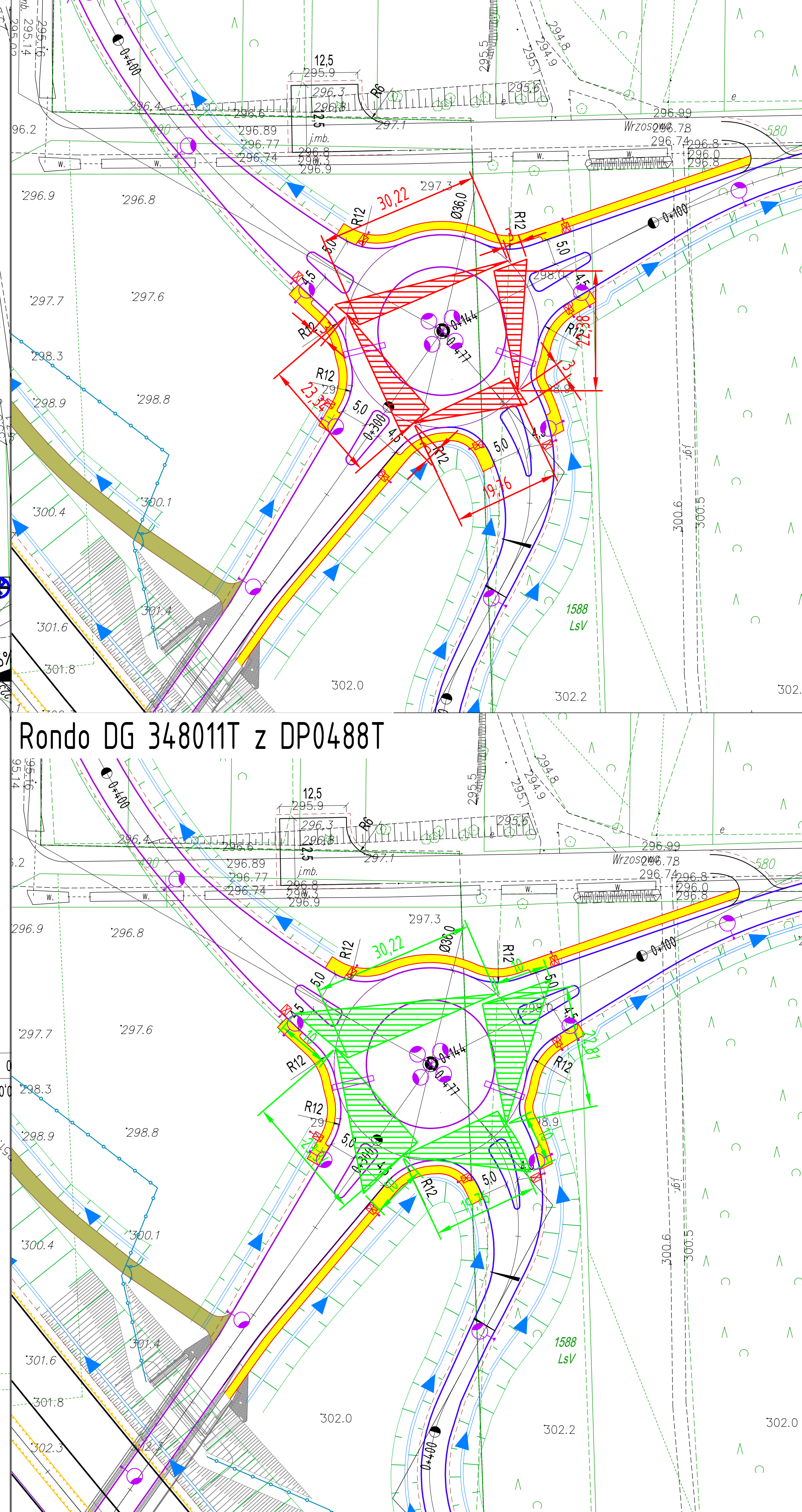
Rondo DG 348011T z DP0488T
